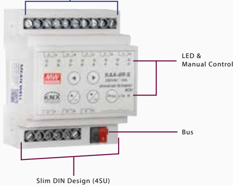
KAA-8R-S W70x H90x D57mm
